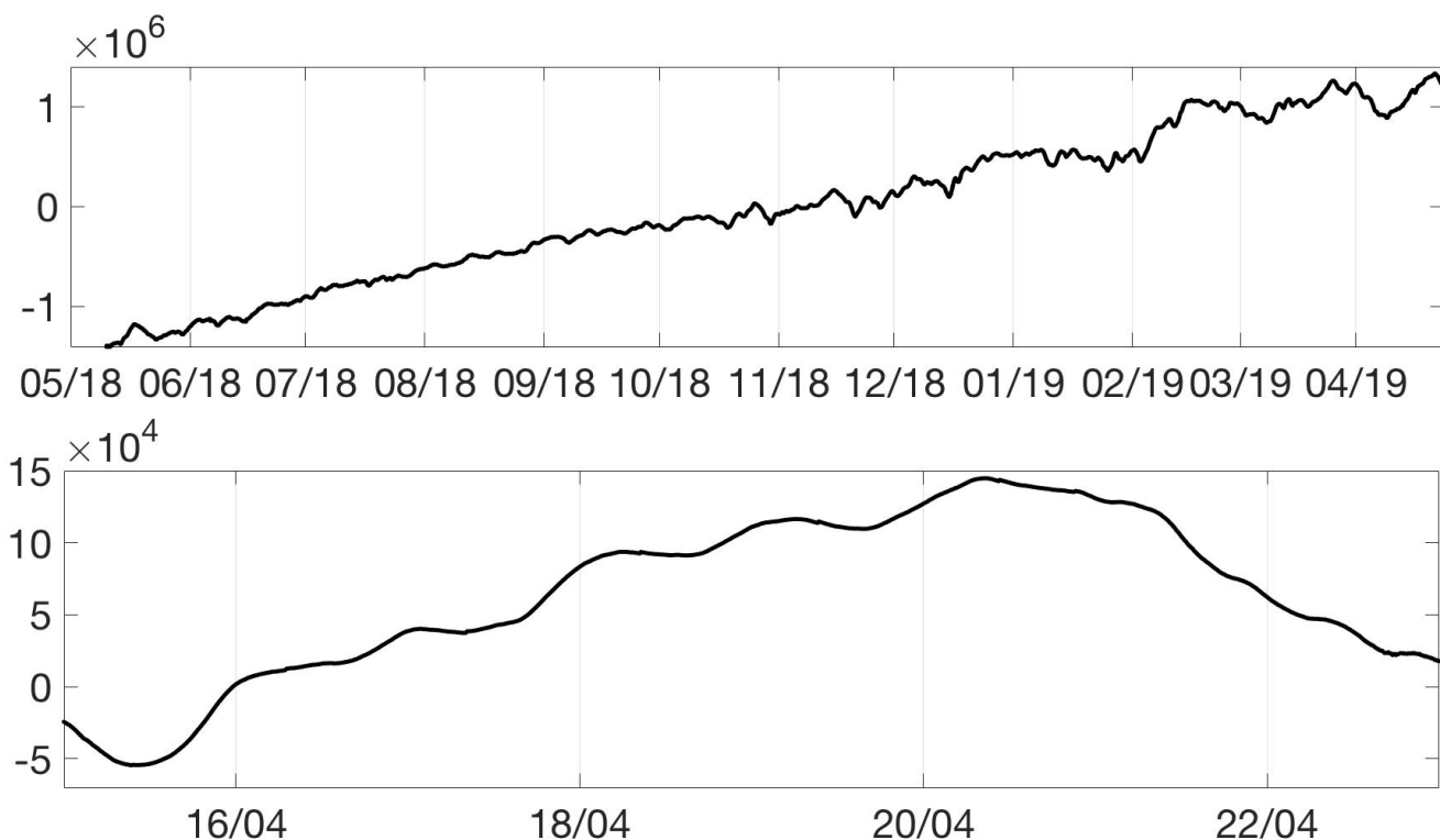
Fig. 4.4 - Grafico relativo ai dati dilatometrici registrati a SVO: in alto viene mostrato lo strain registrato da maggio 2018, mentre in basso quello nell'ultima settimana.
