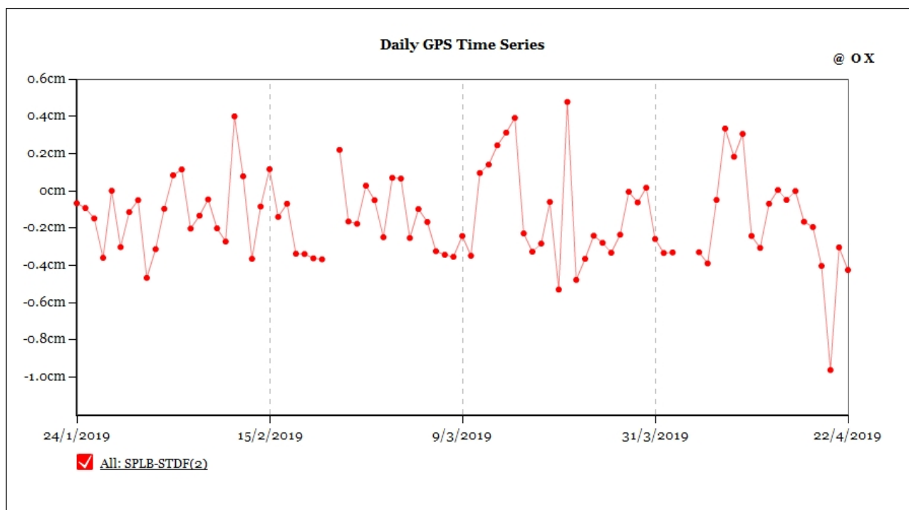
Fig. 5.1 - Serie temporale della variazione di distanza tra STDF (Timpone del Fuoco) e SPLB (Punta Labronzo)
